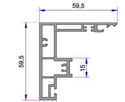
Üç Bölmeli Sürme Alm. Orta Kayıt Profili Profil YENİ Yapılacak
