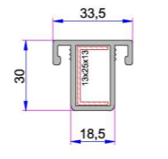
Sürme Sineklik Orta Kayıt Profili P.A.242.3200.600.0.00.01
