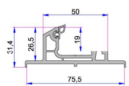
Çift Ray Adaptör Profili P.A.232.5800.600.0.BC.19
