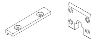
Sürme Üst Yatak Parçası 34009 - 36010
