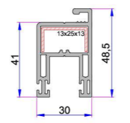
Sürme Sineklik Kanat Profili P.A.242.2305.600.0.00.01
