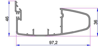
Alm. Kanat Arka Kapama Griyaj Profili 16028.601.5.2.0.9016
