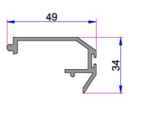
Alm. Kasa Kanal Kapama Profili AD 16 - 013
