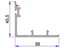
PVC Kanat Ara Bindirme Contası P.A.232.5700.600.0.00.01
