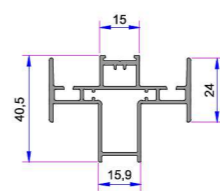
Alm. Kulaklı Çift Kanat Adaptörü Profil YENİ Yapılacak
