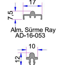
Alm. Sürme Ray AD16-053
