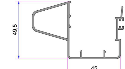
Alm. Kanat Arka Kapama Griyaj Profili Kalıp Yeni Yapılacak
