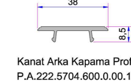
Alm. Kanat Arka Kapama Griyaj Profili Kalıp Yeni Yapılacak
