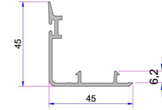
Süper Kanat Arka Kapama Profili P.A.222.5700.600.0.00.19
