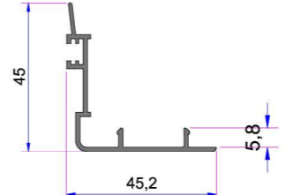
Alm. Süper Kanat Arka Kapama Profili AD16-032
