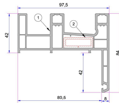
Sineklikli Sürme Kanat Kapama P.A.242.5701.650.0.00.19
